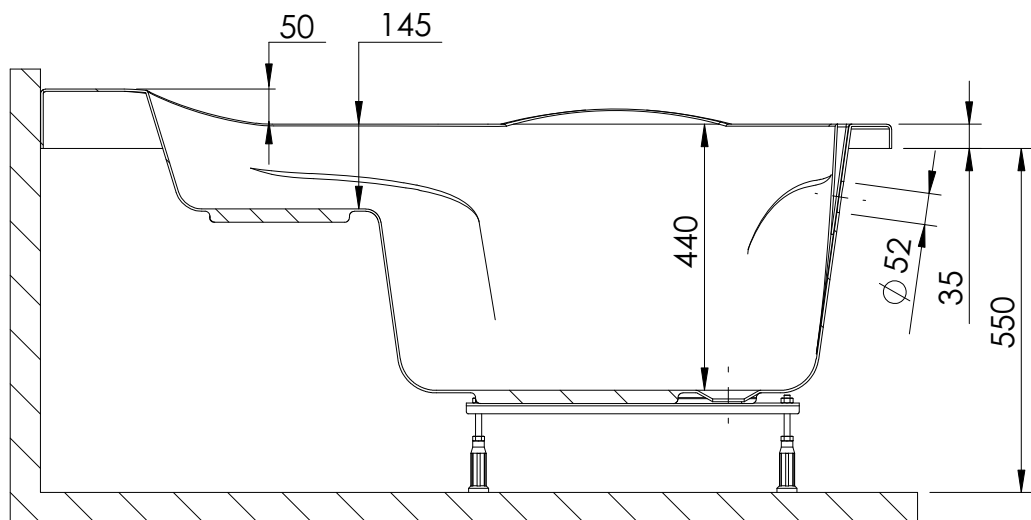
PRZEKRÓJ A-A pojemność: 180 l
