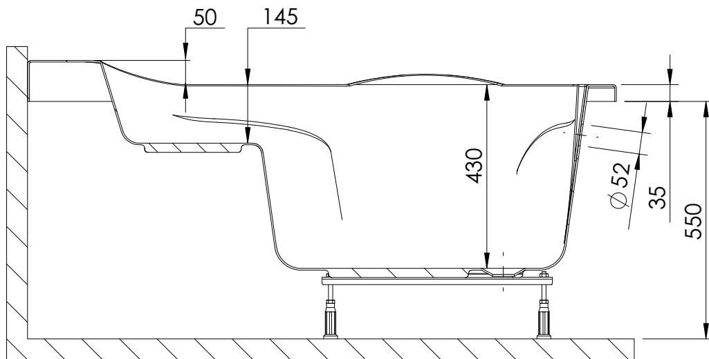
PRZEKRÓJ A-A pojemność: 160 l
