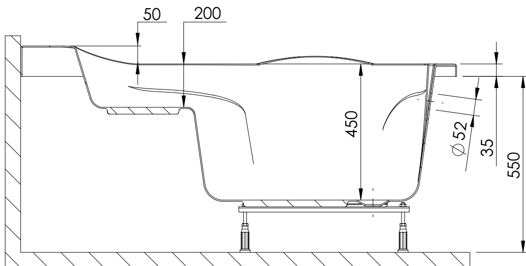
PRZEKRÓJ A-A pojemność: 205 l
