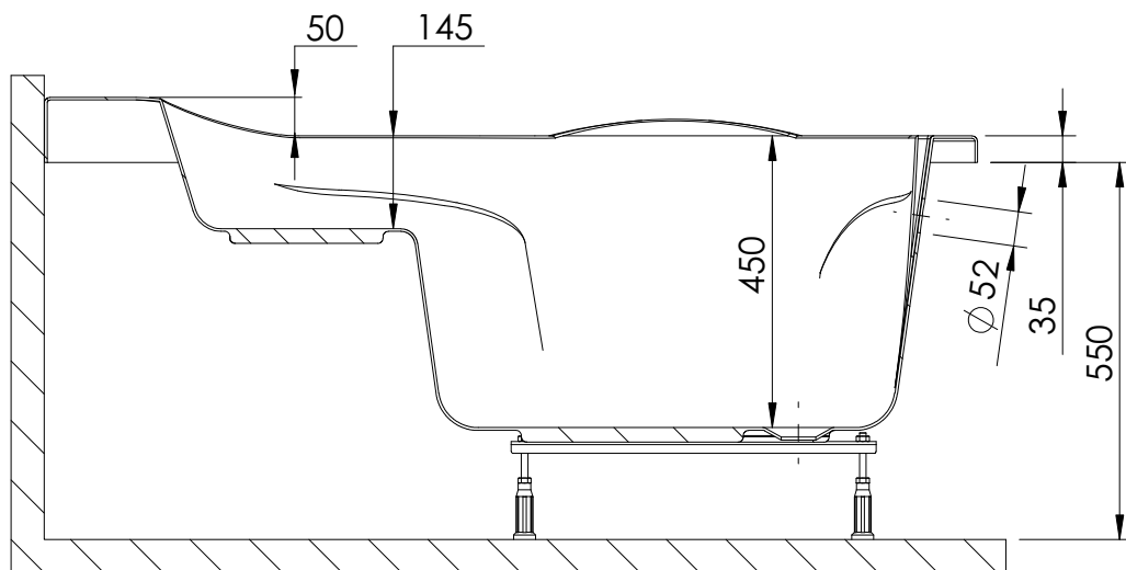
PRZEKRÓJ A-A pojemność: 210 l
