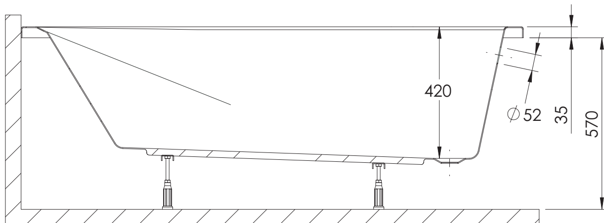
PRZEKRÓJ A-A
