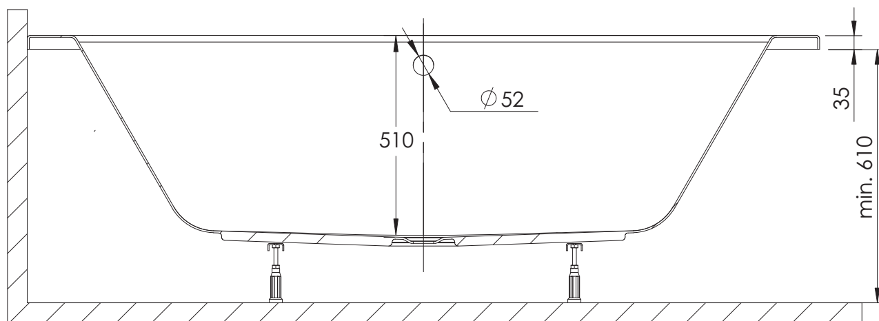
PRZEKRÓJ A-A
