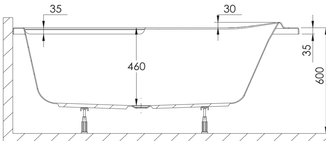
PRZEKRÓJ A-A
