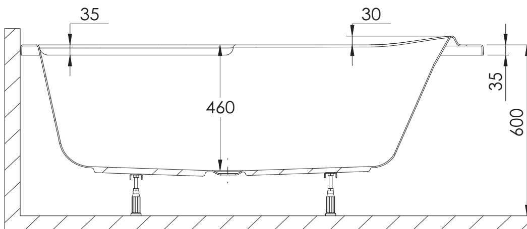
PRZEKRÓJ A-A
